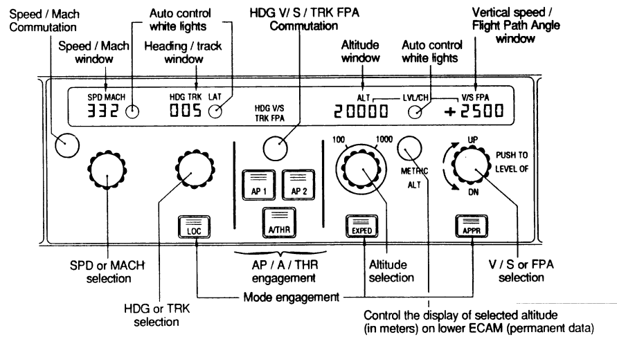
Airbus A320
